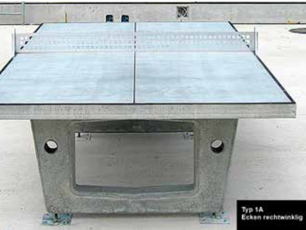
Fig. type 1A Coins à angle droit
