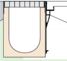
Finition sur caniveau de drainage
