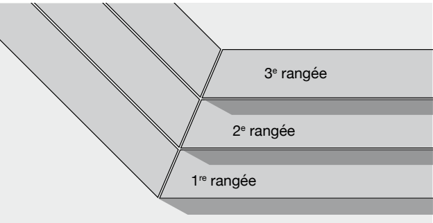
Coin 45°, avec éléments spéciaux (sur commande)
