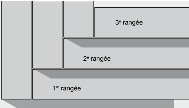
Coin 90°, avec éléments normaux et de finition
