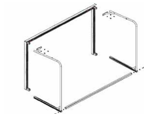
But de handball „Zerlegbar“
